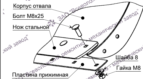
Рис.5 Крепление ножа
