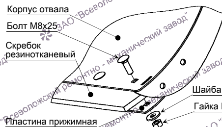
Рис.6 Крепление скребка
