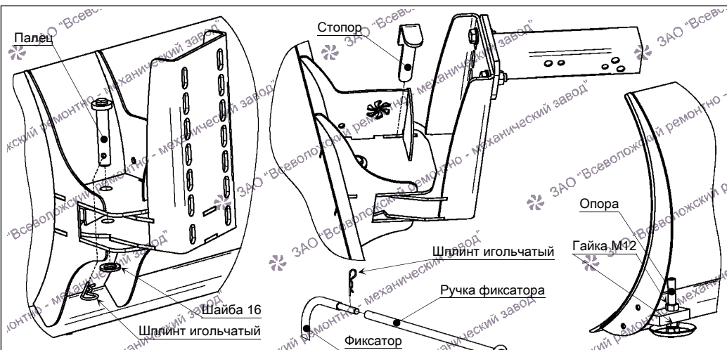
Рис.1 Установка пальца
