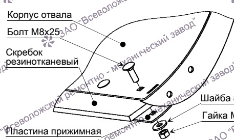
Рис.6 Крепление скребка
